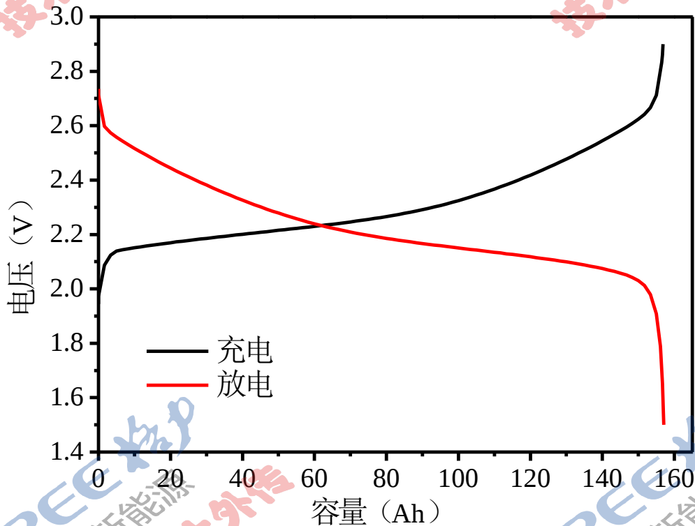
图一 常温 1C 充放电性能曲线图
